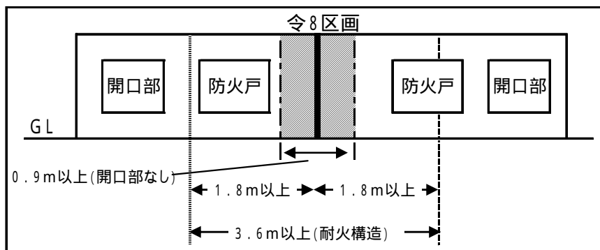
《突き出しを設けずに縦に令8区画した例》
