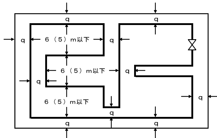
一辺省略と二辺省略の組合せの例
