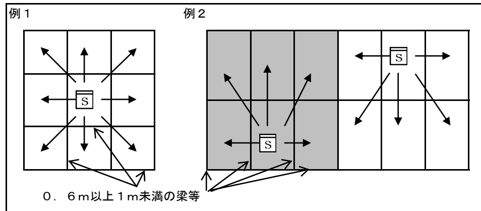
《同一の感知区域とすることができる場合の例》
